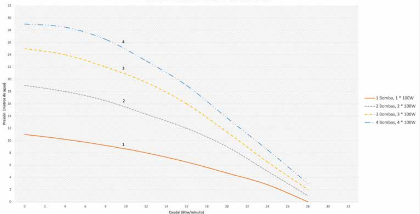
Bombas ZL50 en serie con panel solar de 100 Wp
